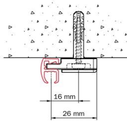
Montage au plafond avec support plafond 2150.
