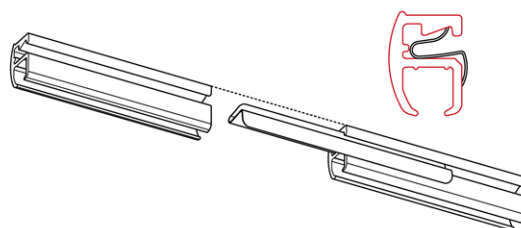
2152 Connecteur de rail Application de connecteurs de rail métalliques au dos du 2102.
