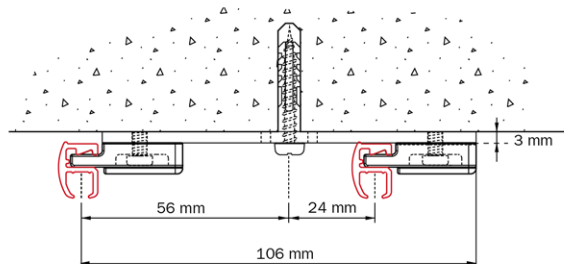
Pour une installation parfaitement parallèle : montage avec support double 2216 et supports plafond 2150.
