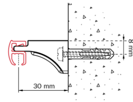
Montage au mur avec support mural 2151.
