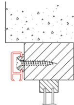
Montage sur chambranle avec le 2254.
