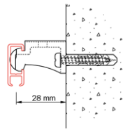
Montage au mur avec le 2251.
