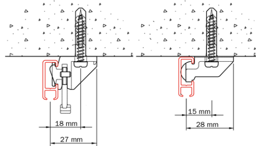
Montage au plafond avec le 7450.
