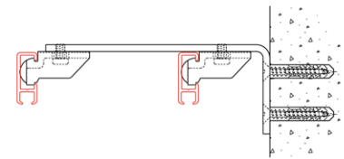
Montage au mur avec le support mural 2015.
