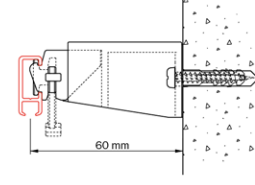
Montage au mur avec le 7451.
