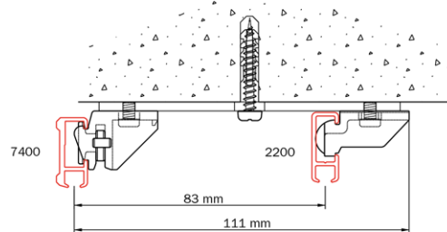
Montage au plafond avec le 2216 & 7450 resp. 2250.
