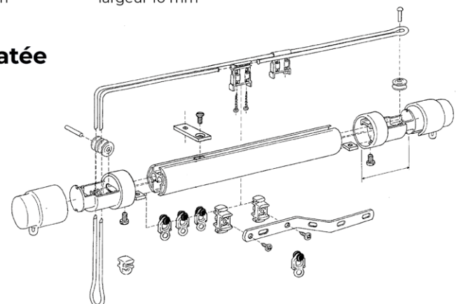
Tête de rideau avec glisseur décalé 6010 largeur 15 mm
