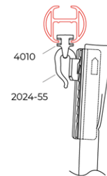
sans tête de rideau avec glisseur 4010 largeur 10 mm
