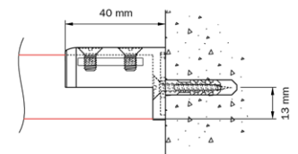
Montage au mural 5100 avec naissance 5149
