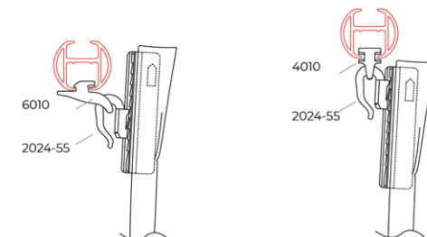
Tête de rideau avec glisseur décalé 6010 largeur 15 mm
