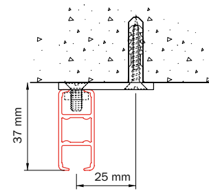
Montage au plafond avec support plafond 4135
