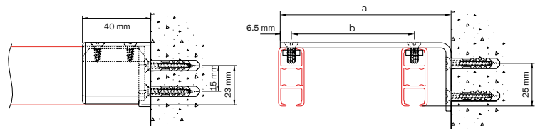
Montage au mur avec support 4149
