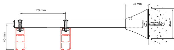
Montage avec équerre réglable 4217
