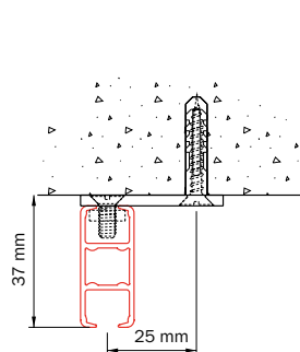
montage au plafond 4100 avec support plafond 4135
