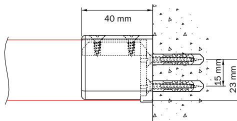
Montage au mural 4100 avec naissance 4149
