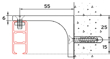
Montage au mural avec support mural 4140
