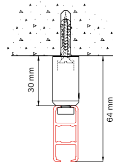
montage au plafond 4100 avec montant de plafond 4254
