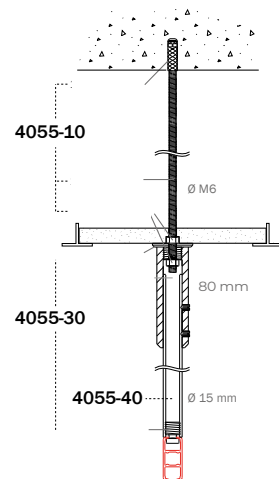
Montage au plafond 4100 sur un pied 4055-40 avec kit de montage 4055-10, pied avec extrémité fileté 4055-30.
