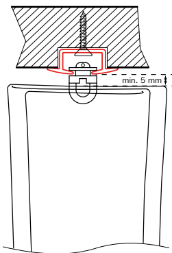
Rideau suspendu sous le rail
