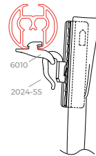
Tête de rideau avec glisseur décalé 6010 largeur 15 mm
