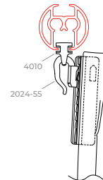
sans tête de rideau avec glisseur 4010 largeur 10 mm
