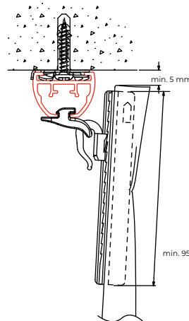
5600 avec tête de rideau avec 6010 glisseur
