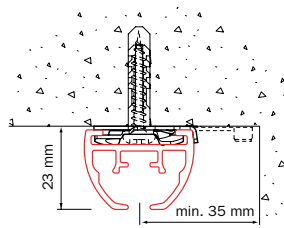
Montage au plafond avec bride 6050
