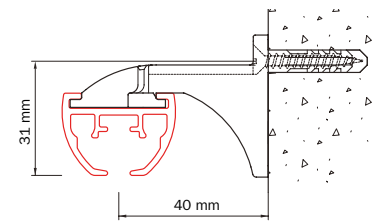
Montage au mural avec support mural 6051
