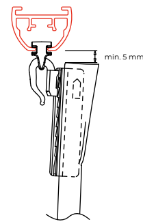
5600 sans tête de rideau avec 4010 glisseur
