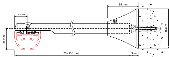
Montage au mur avec support recoupable 6017
