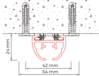
Montage au plafond avec support plafond 6055-1000
