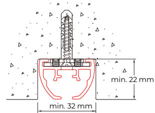
Montage à l'aveugle par exemple dans une rainure avec support 6055-3100-N-040 pour les courbes : fraiser une rainure sur la base du rail livré. Préperforation en usine par Qurails.
